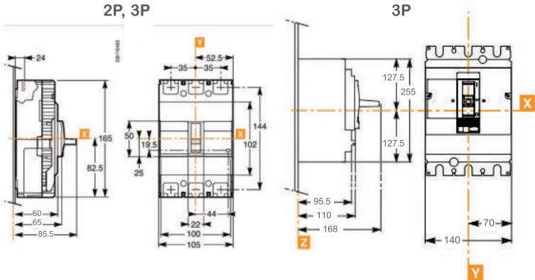
Kích thước EYC250
