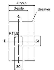
Front-panel cutout
